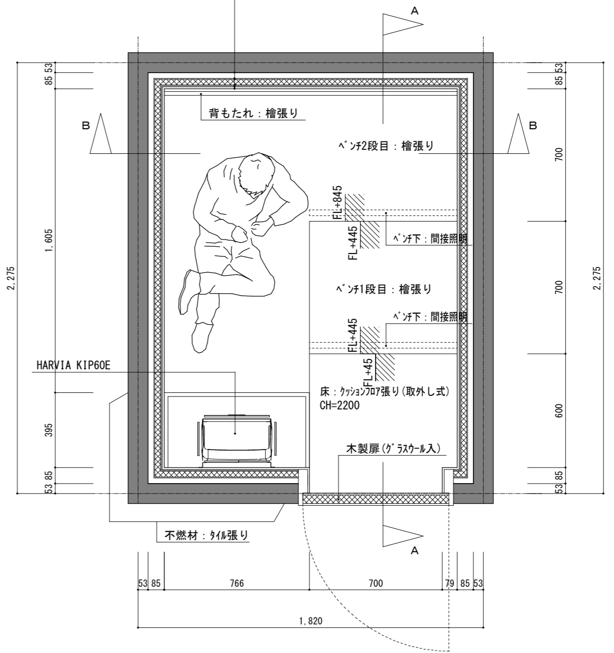
1620L型サウナ室平面図 S=1/20
